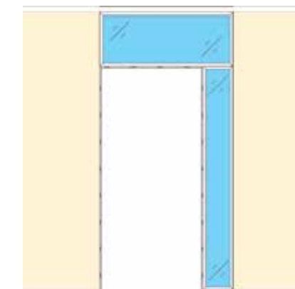
⑰ BEGLAASD BOVEN- EN ZIJLICHT voor enkele deur
